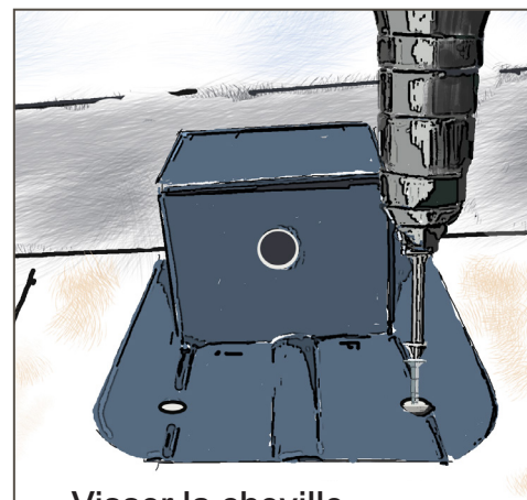
Visser la cheville 2 chevilles par platine
