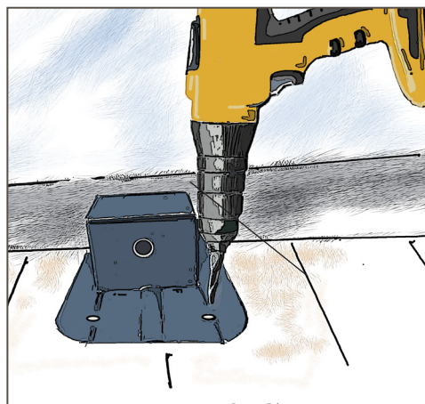
Perçage Forêt Ø5 2 perçages par platine
